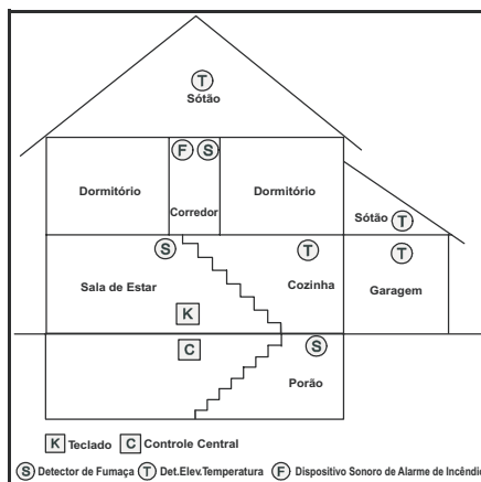
FIGURA 3: Instalação Típica de Alarme de Incêndio
